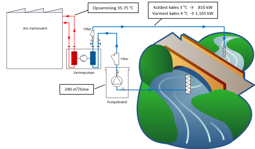
Figur 7.4 – Principdiagram for varmepumpe i Ans. Kilde: Teknologisk Institut.
