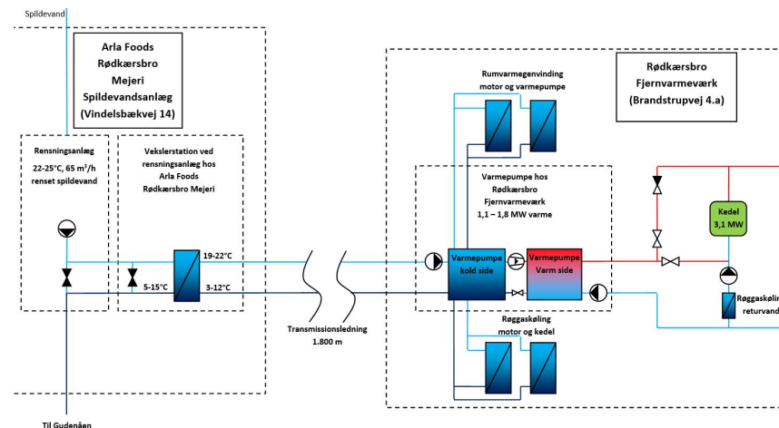
Figur 5.2 – Varmepumpeanlægget i Rødkærsgro. Til venstre ses spildevandsledningen som løber til Gudenåen men ledes igennem pladevarmevekslerne for det uddledes. Varmepumpen er installeret på varmeværket omkring 1800 m fra rensningsanlægget. Varmevækslerne til øget røggaskøling nederst på figuren er ikke installerede.
