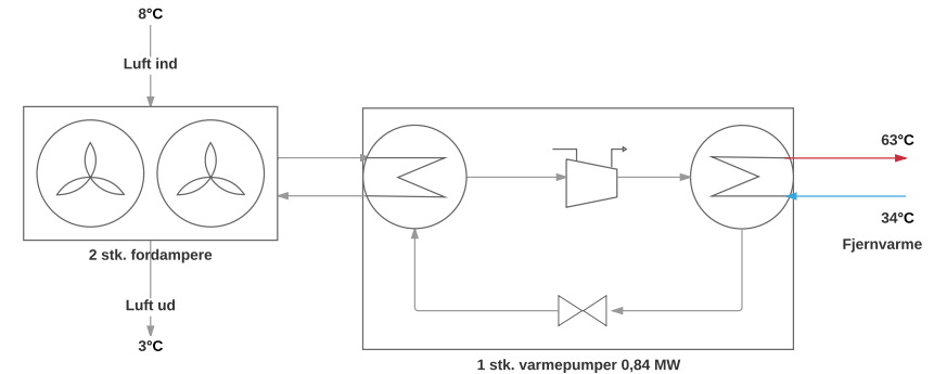
Figur 8.6 – Principskitse af el-drevet varmpumpe koblet til luftkølere.
