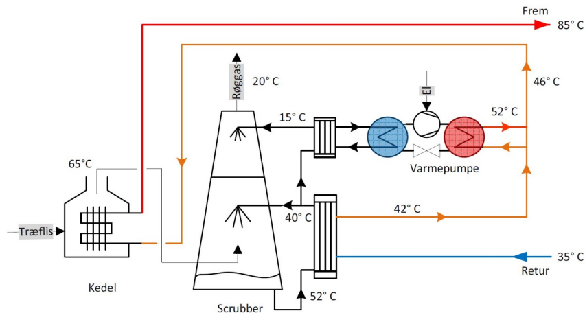
Figur 2.9 – Principskitse af eldrevet varmepumpe koblet til scrubbertårn på flis kedel. Kilde: Teknologisk Institut.
