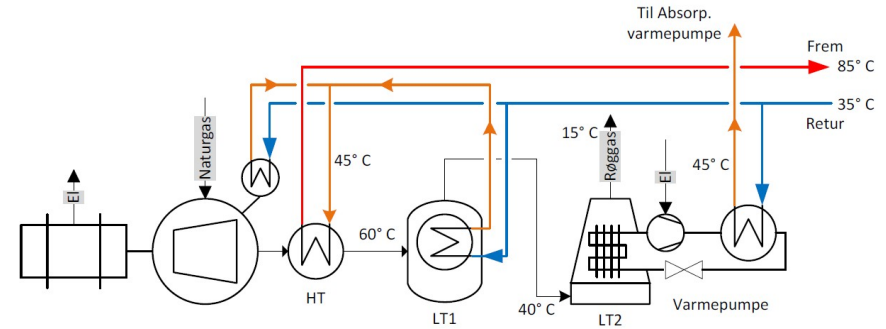
Figur 2.5 – Principskitse af eldrevet varmpumpe til røggaskondensering på motoranlæg. Kilde: Teknologisk Institut.
