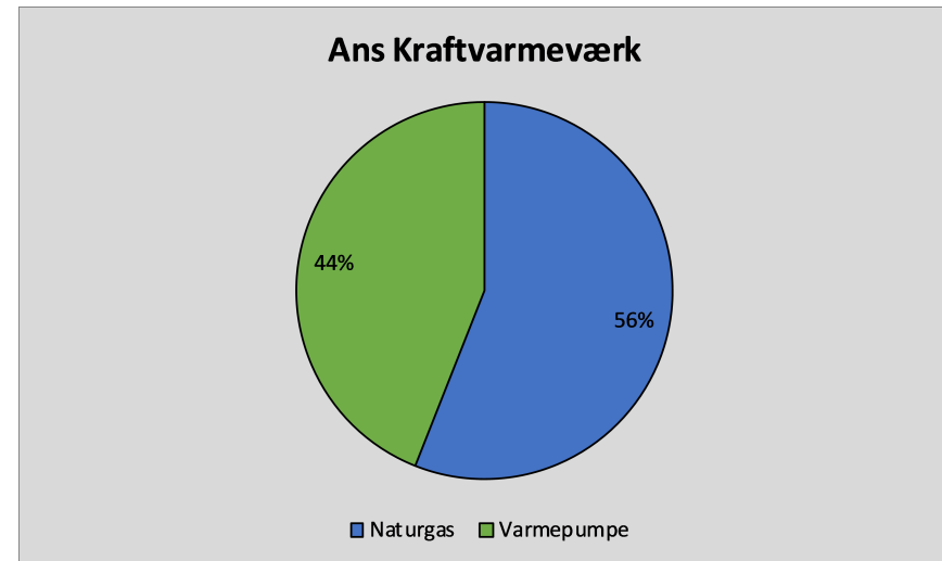
Figur 7.2 – Forventet varmeproduktionsfordeling ved Ans Kraftvarmeværk med varmepumper.
