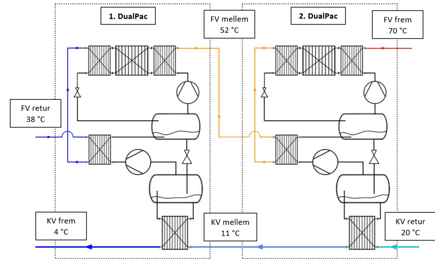
Figur 5.3 – Principskitse over spildevandsvarmepumpen i Rødkærsbro.
