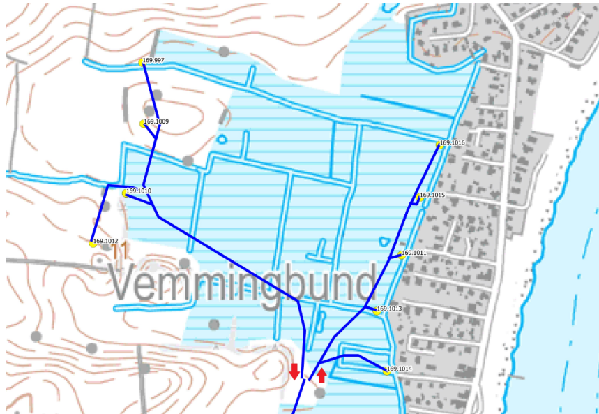
Figur 6.7 – Placering af indvindingsboringer (tv.) set i forhold til injektionsboringer (th.) Helt til højre ses Vemmingbund der støder ud til Sønderborg Bugt og Flensborg Fjord.
