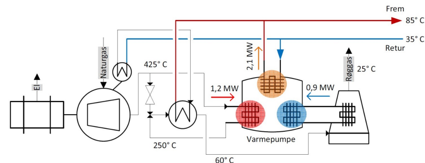
Figur 2.2 – Principskitse over absorptions-varmpumpe til røggaskondensering på motoranlæg. Kilde: Teknologisk Institut.
