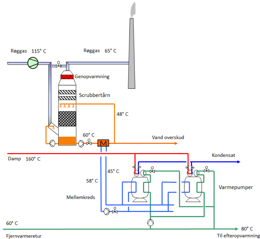
Figur 2.11 – Principskitse over absorptions-varmpumper ved Vestforbrænding. Kilde: Vestforbrænding.
